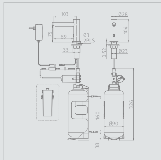
Metrix Seifenspender 1991010 | 1991023
