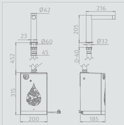
Metrix Handtrockner 1990201
